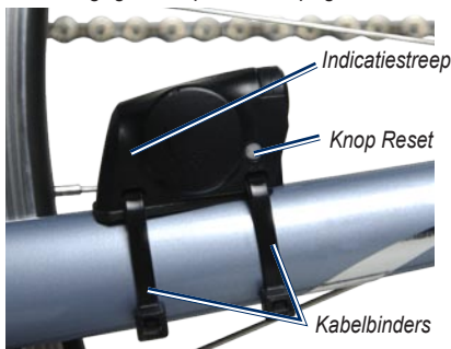
GSC 10 op achtervork
