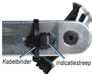
Pedaalmagneet op hefboom
