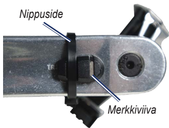
Poljinmagneetti poljinkammessa
