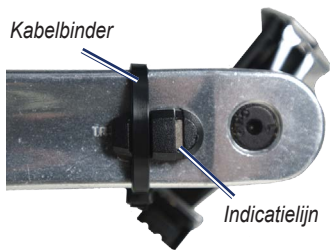
Pedaalmagneet op trapperarm
