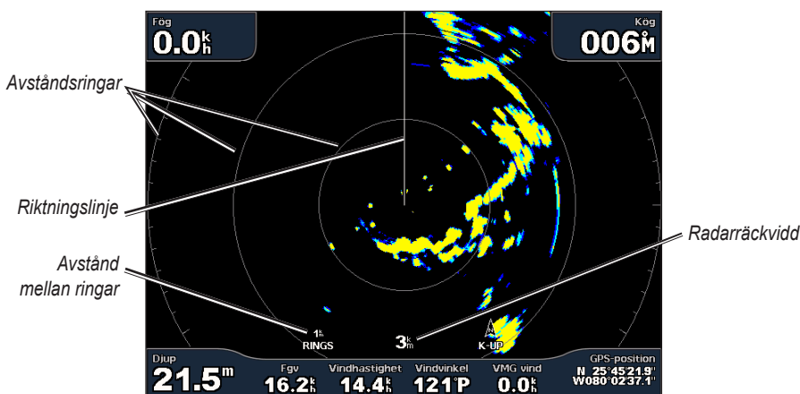
Navigationläge
