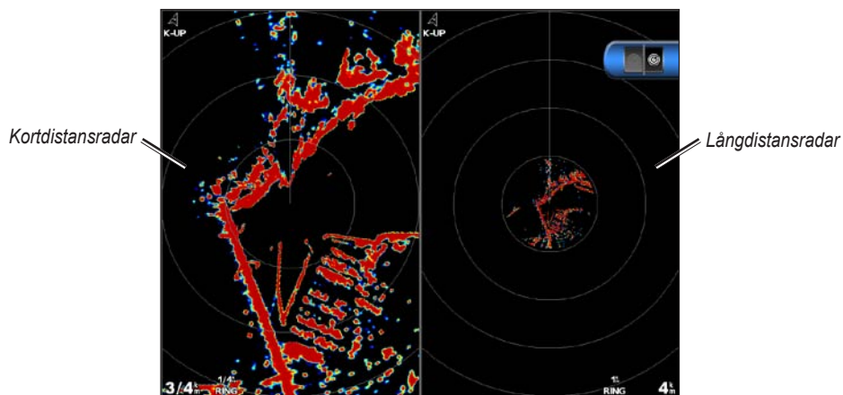
Dubbelt mätområdesläge
