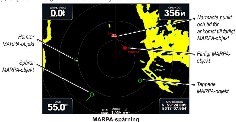
MARPA-spårning
