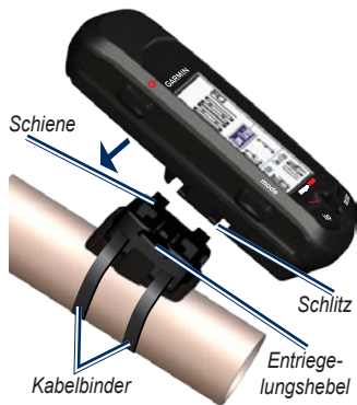
Draufsicht des Edge bei der Montage auf eine horizontale Stange
